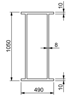
Mặt cắt dầm chính
